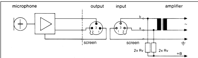
Fig. 5: branchement avec un transformateur d'entrée sans prise centrale (sans mise à la terre)
